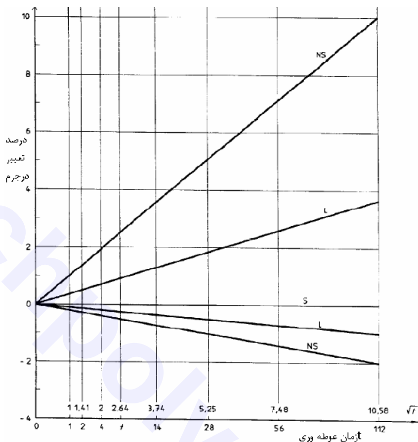
شکل ۱- نمودار طبقه بندی لوله های PVC-C ، PVCHI و PVC-U بر اساس تغییر در جرم
