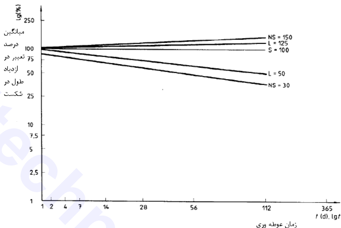
شکل ۴- نمودار طبقه بندی برای لوله های PVCHI, PVCU و PVCC بر اساس درصد تغییر در ازدیاد طول در شکست
