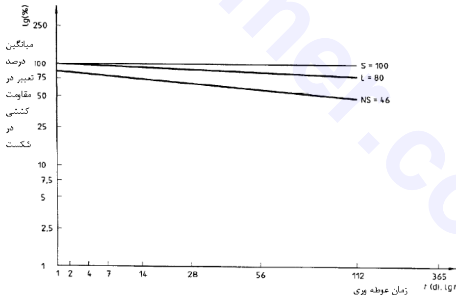
شکل ۳- نمودار طبقه بندی برای لوله های PVC-U, PVC-HI و PVC-C بر اساس درصد تغییر استحکام کششی در شکست
