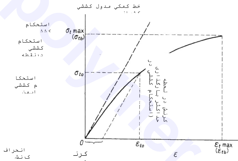
شکل 2- پ - منحنی تنش- کرنش کششی (مدل 3)
