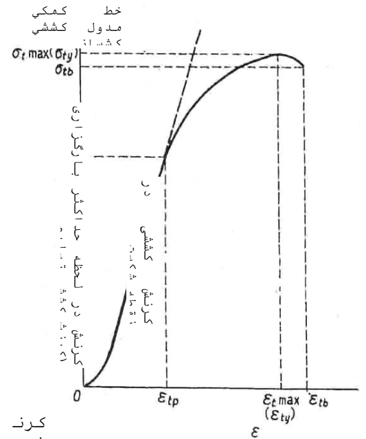
شکل 2- الف- منحنی تنش-کرنش کششی (مدل 1)
